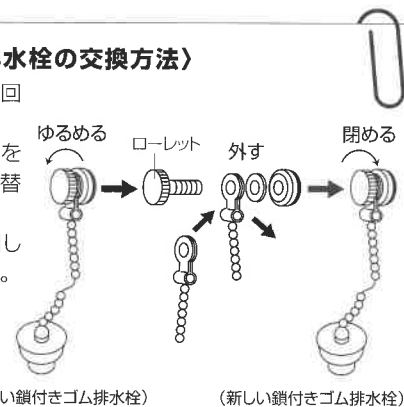
(古い鎖付きゴム排水栓)
